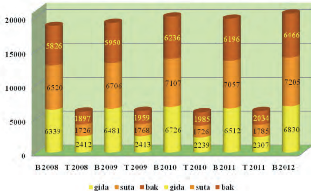
1. ábra: Őz létszámbecslés (B) és teríték (T) Pest megyében 2008-2012.
