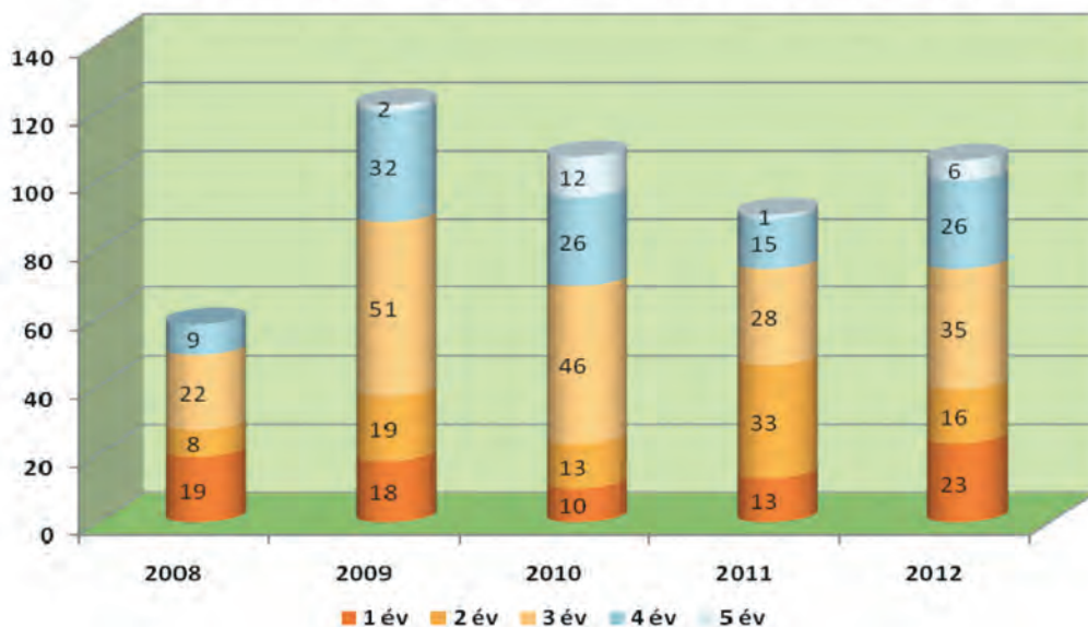
6. ábra: A minuszpontos őzbakok kormegoszlása 2008-2012. (10. 25-ig)
