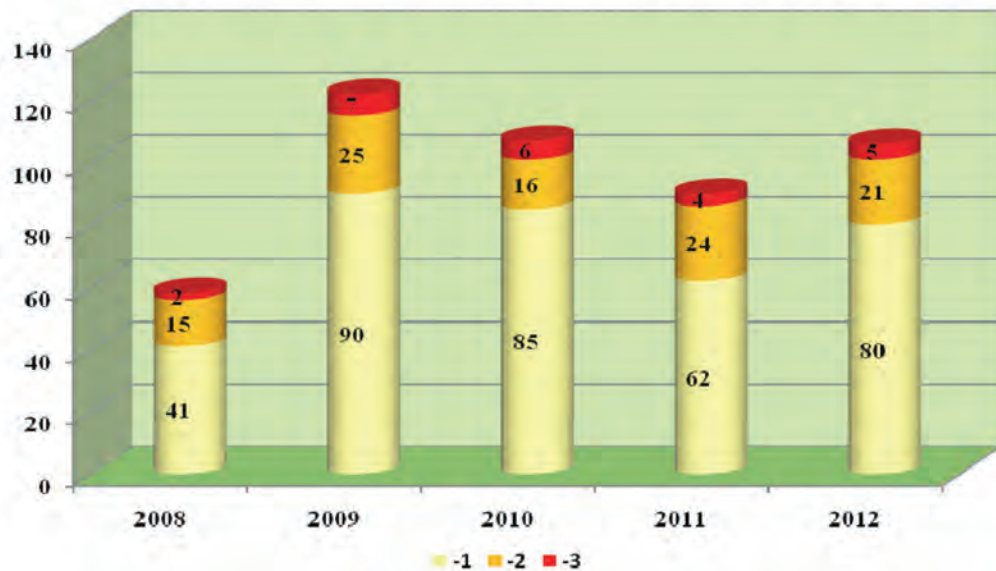
5. ábra: Minuszpontos őztrófeák Pest megyében 2008-2012. (10. 25-ig)
