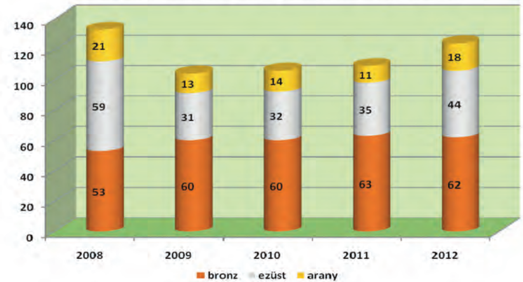
3. ábra: Érmes őztrófeák Pest megyében 2008-2012. (10. 25-ig)
