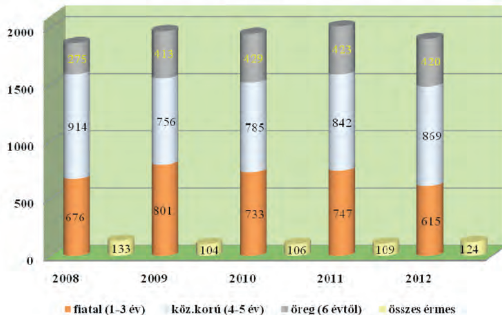
2. ábra: Elbírált bakok korosztályi megoszlása Pest megyében 2008-2012. (10. 25-ig)
