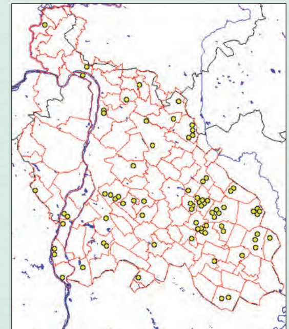
4. ábra: A 2008–2012 között ejtett aranyérmes bakok vadászterületek közötti megoszlása Pest megyében
